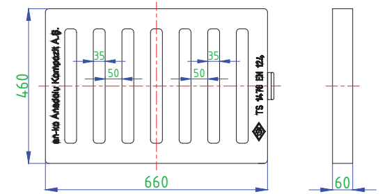
ANKO-GG-207 Yağmur Suyu Izgara (460 x 660 mm)
