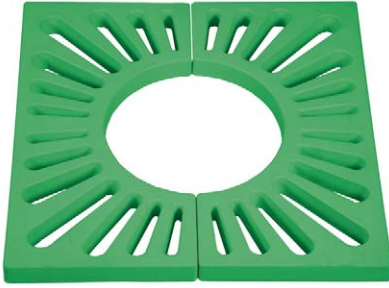
ANKO-TG-103 Ağaç Dibi Izgara (800 x 800 mm) Tip : 4 Parçalı Ağırlık : 8 kg
