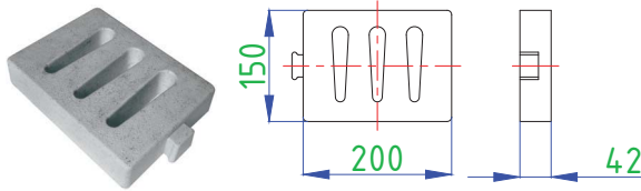
ANKO-TG-201 Ağaç Dibi Izgara Adaptör (600 x 600 mm)
