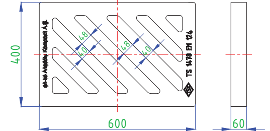
ANKO-GG-203 Yağmur Suyu Izgara (400 x 600 mm)
