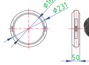
ANKO LA 200 Direk Altı Kelepçe (12 m)
