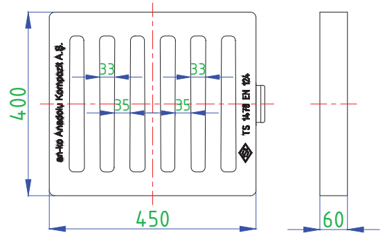
ANKO-GG-206 Yağmur Suyu Izgara (400 x 450 mm)
