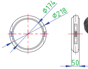
ANKO-LA-100 Direk Altı Kelepçe (10 m)
