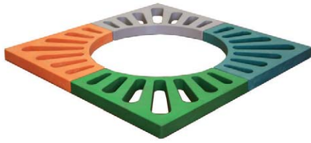
ANKO-TG-102 Ağaç Dibi Izgara (1000 x 1000 mm) Tip : 4 Parçalı Ağırlık : 14 kg
